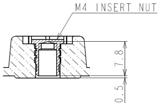
INSERT NUT 断面
