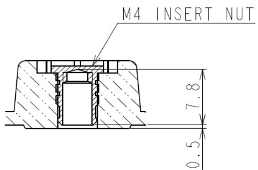
INSERT NUT 断面
